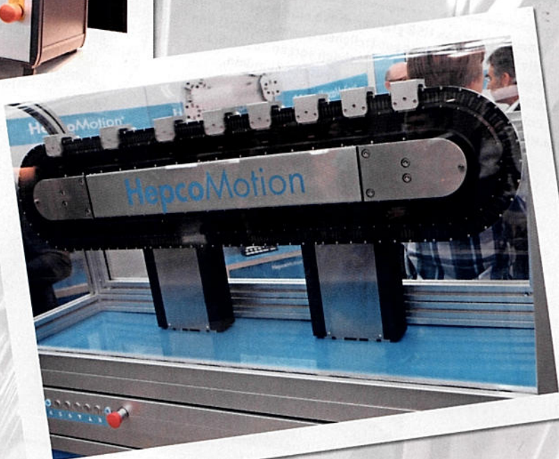
Hepco Motion hat u. a. sein Führungssystem 1-Trak und das XTS von Beckhoff in einem System vereint. So führen die 1-Trak-Linearführungen die sogenannten Mover des linearen Transportsystems XTS von Beckhoff.
